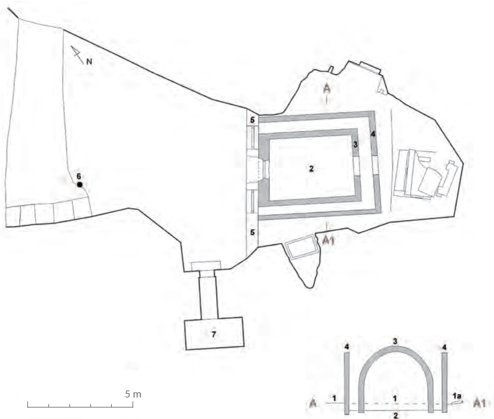
Sl. 56. Gore: tlocrt špilje sv. Ante i terase ispred špilje; dolje: poprečni presjek bunkera. 1) razina poda crkve; 1a) očuvani segment popločenja; 2) betonski pod bunkera; 3) i 4) zidovi bunkera; 5) pročelni zid crkve; 6) urezani natpis 1936 na betonskom ojačanju ogradnog zida terase; 7) prostorija izdubljena u stijeni (crtež: E. Podrug, M. Rak; podloga: Geodetska mjerenja d.o.o.).
