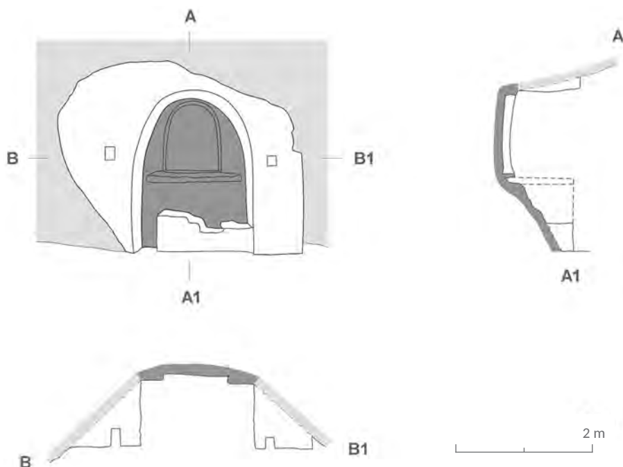
Sl. 38. Bočni oltar: nacrt i presjeci. Sjenčano sivo: prirodna površina matične stijene; sjenčano tamnosivo: obrađena pritesana površina matične stijene (crtež: E. Podrug, M. Rak).
